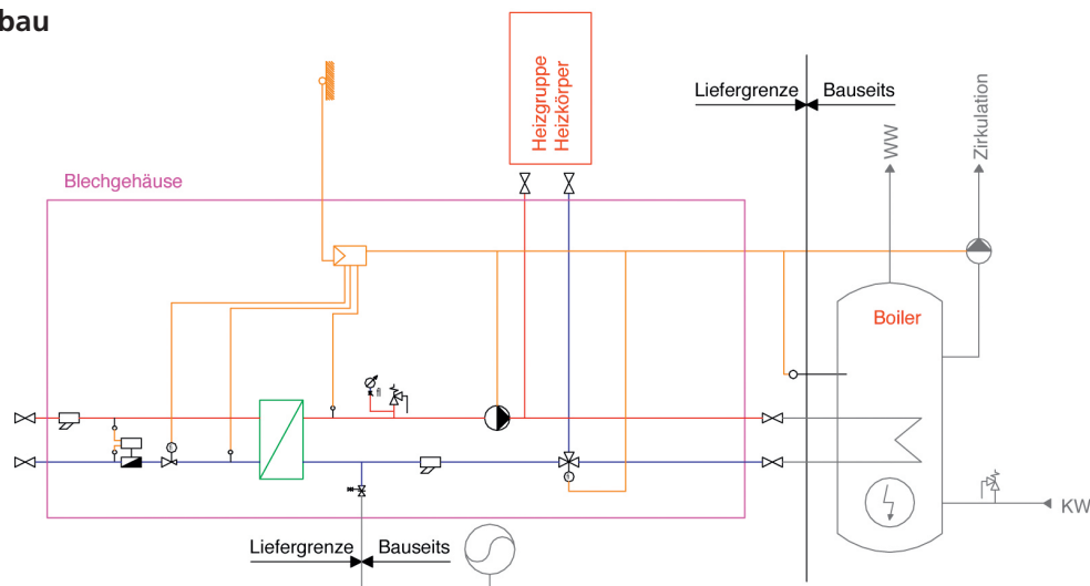
Grundstation
